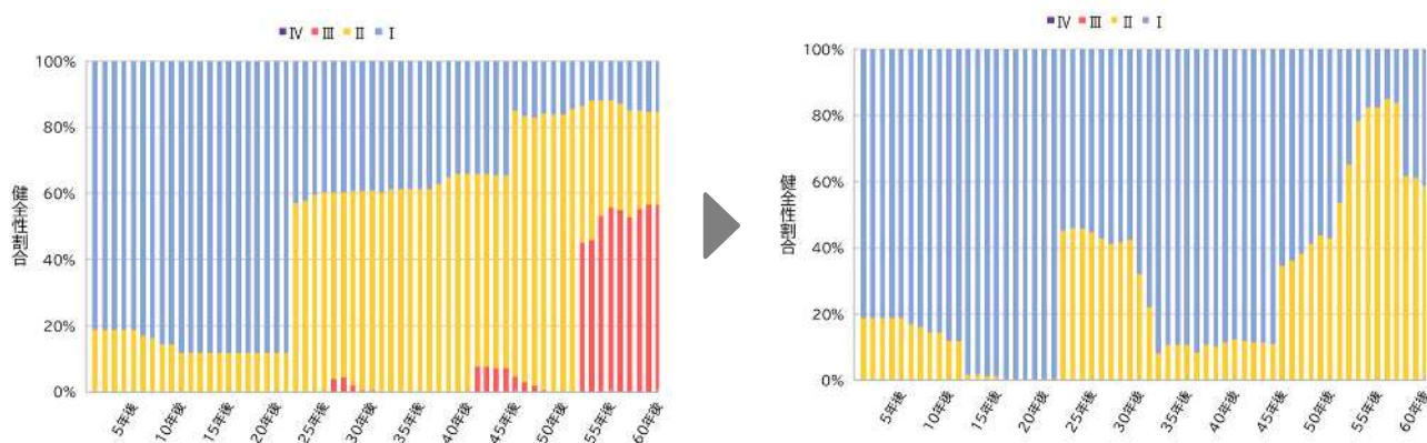
図-3.5 健全性の推移（左：事後保全型、右：予防保全型）
